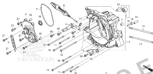
M-19.10 Carcaça do Motor Direita
