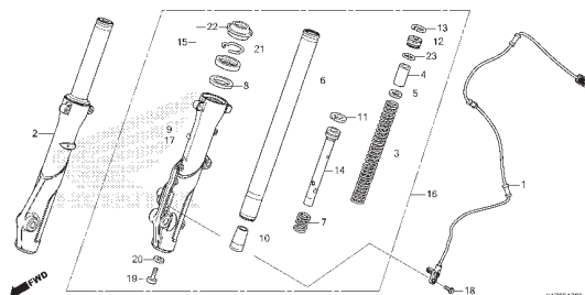
C-17 Garfo Dianteiro
