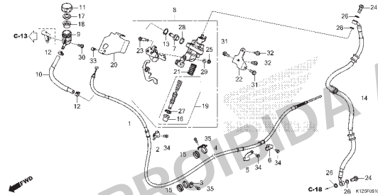
C-5.10 Cilindro Mestre do Freio
