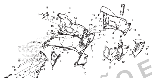
C-15 Tampa da Carcaça
