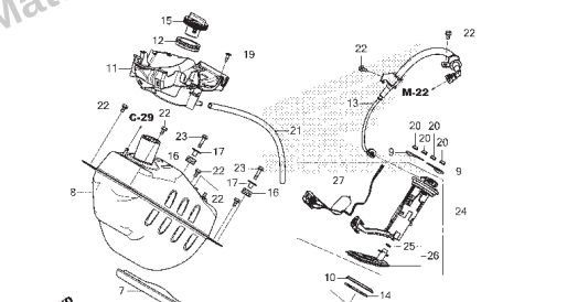
C-26 Tanque de Combustível
