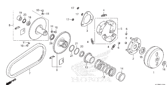
M-17 Flange Movido
