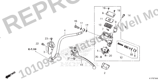
C-6 Cilindro Mestre do Freio Traseiro
