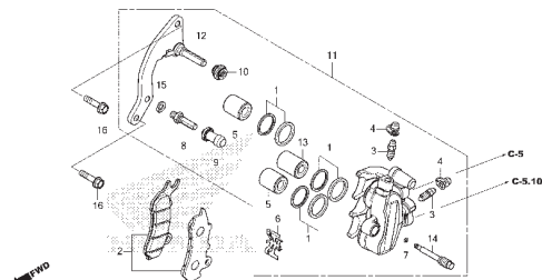
C-21 Cáliber do Freio Traseiro
