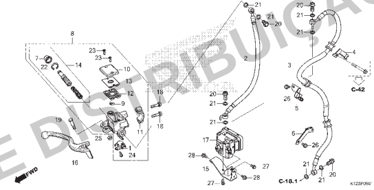
C-7.10 Tubo de Freio Traseiro
