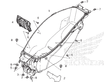
C-16 Compartimento de Bagagem
