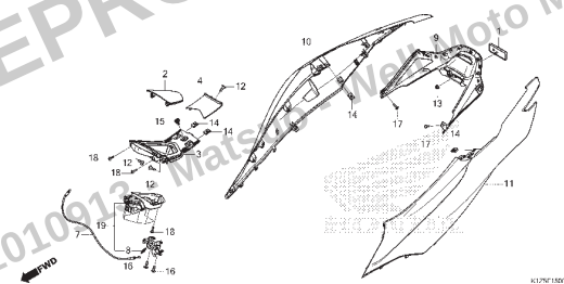
C-15 Tampa da Carcaça
